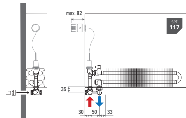
Voorbeeld aansluiting links
