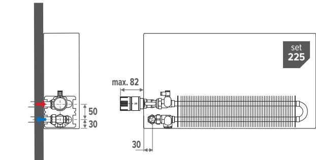
Voorbeeld aansluiting links
