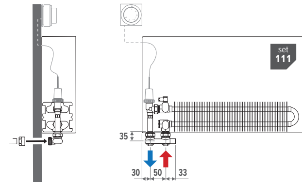
Voorbeeld aansluiting links
