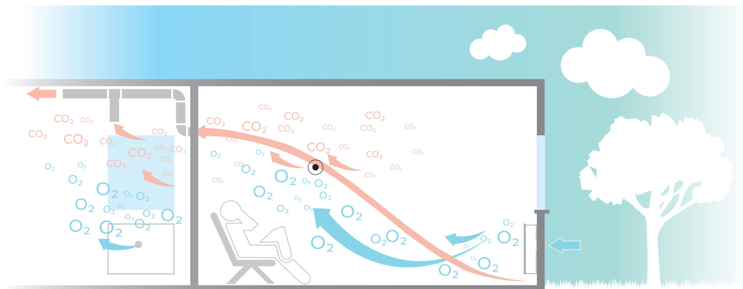
Decentrale luchttoevoer en centrale luchtafvoer
